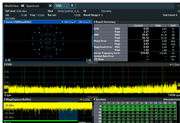
Демодуляция сигнала DVB-SX2 с несколькими модуляциями с помощью опции R&S®FPL1-K70M (требуется опция R&S®FPL1-K70)
