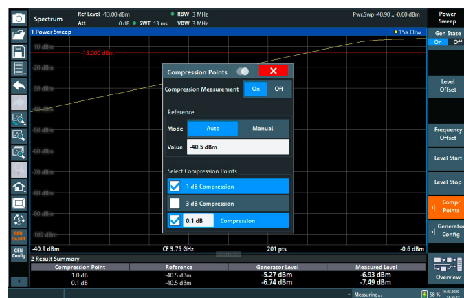
Измерение точек компрессии 1 дБ и 0,1 дБ
