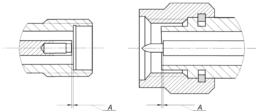
Рисунок 3.4 Соединители тип 3,5 мм и IX (розетка и вилка)
