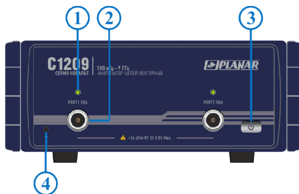
Рисунок 4.5 Передняя панель
