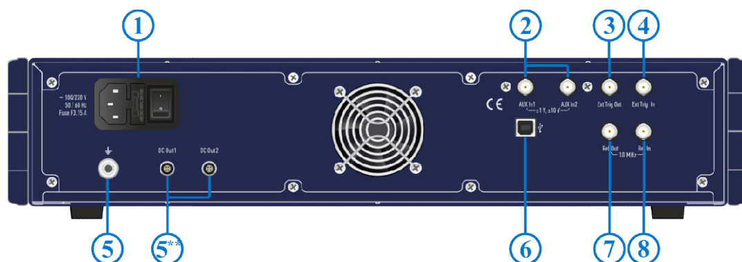
Рисунок 4.24 Задняя панель
