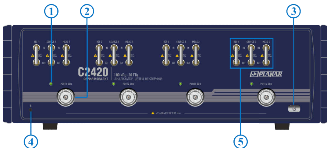
Рисунок 4.21 Передняя панель
