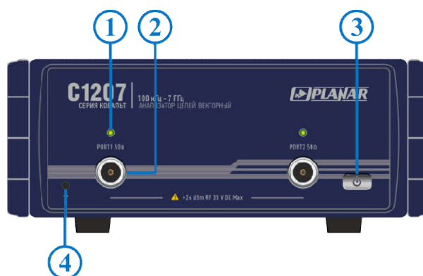
Рисунок 4.3 Передняя панель
