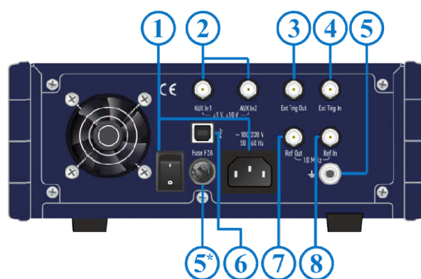
Рисунок 4.2 Задняя панель
