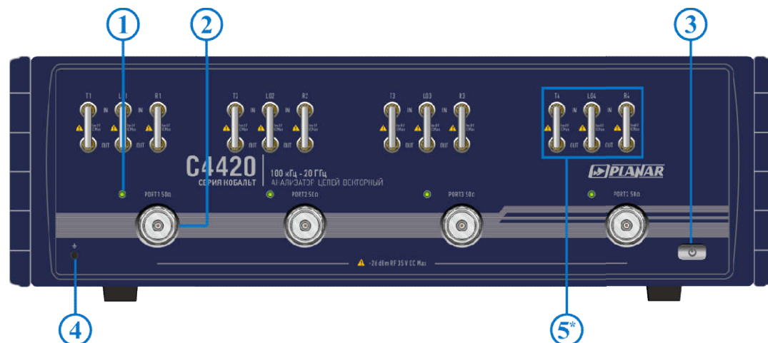
Рисунок 4.29 Передняя панель
