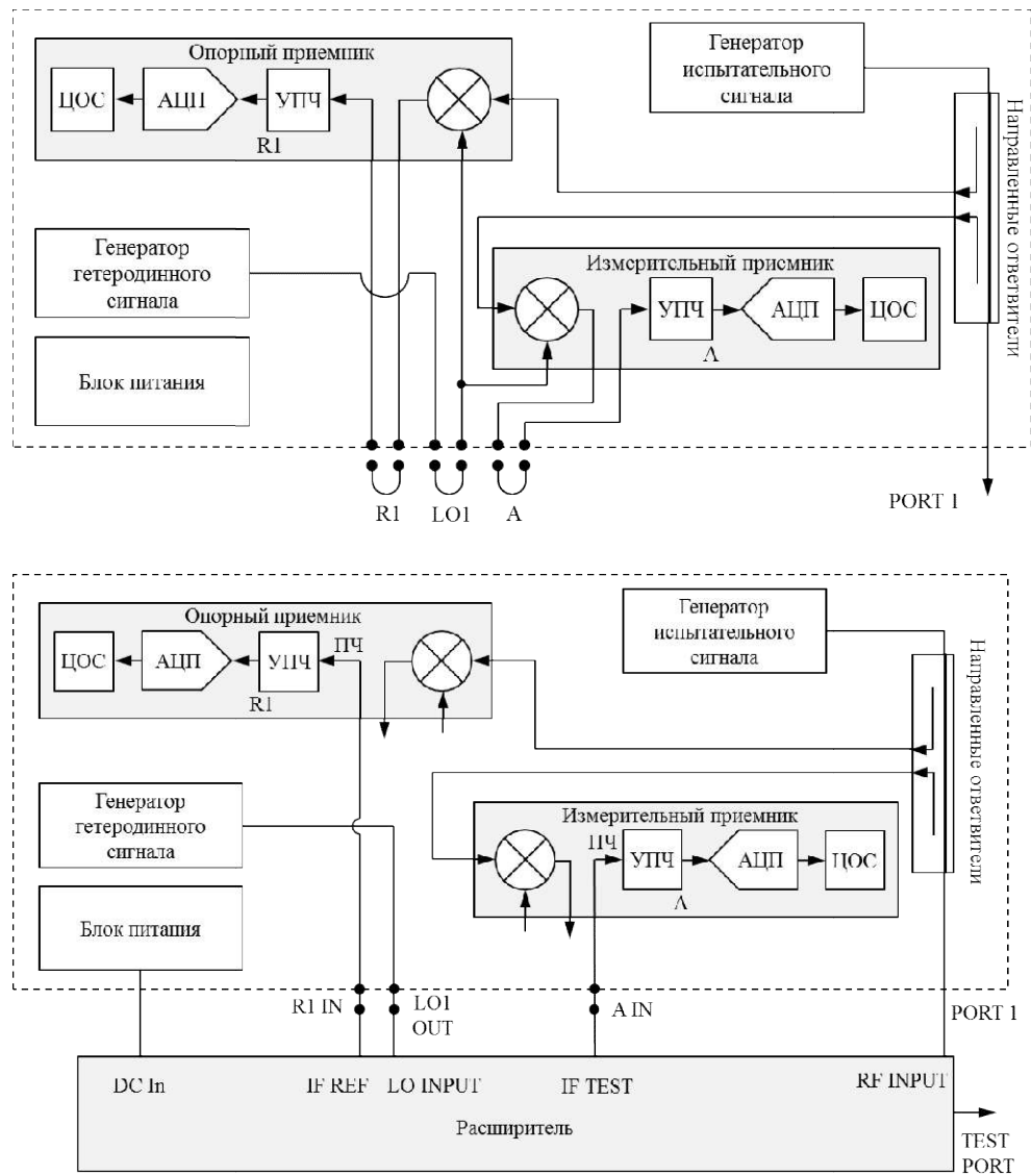
Рисунок 2.5 Подключение расширителя по частоте
