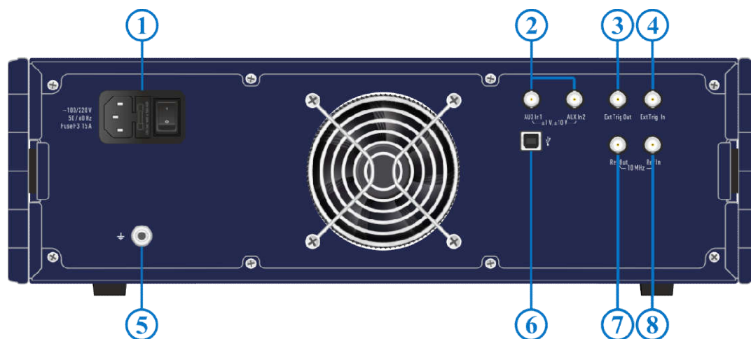
Рисунок 4.8 Задняя панель
