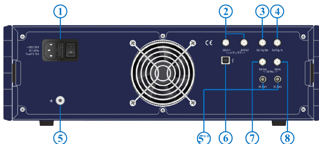
Рисунок 4.28 Задняя панель
