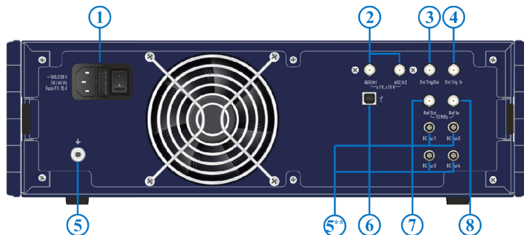
Рисунок 4.30 Задняя панель
