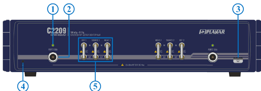
Рисунок 4.15 Передняя панель
