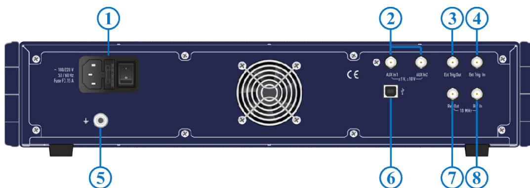
Рисунок 4.12 Задняя панель
