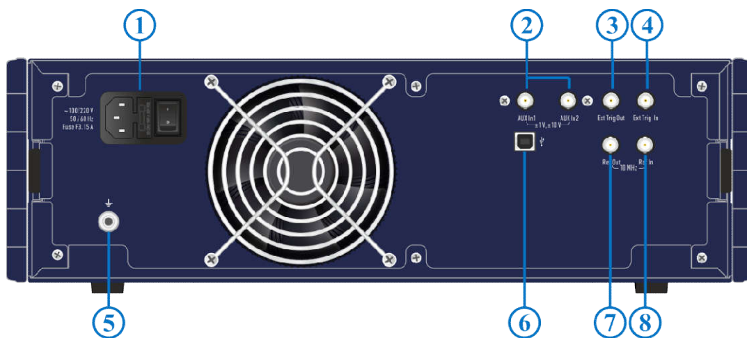
Рисунок 4.22 Задняя панель
