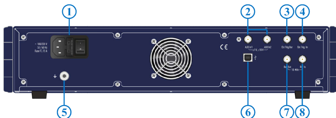
Рисунок 4.16 Задняя панель
