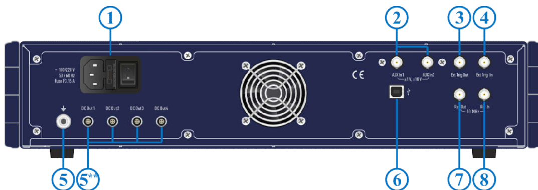
Рисунок 4.26 Задняя панель
