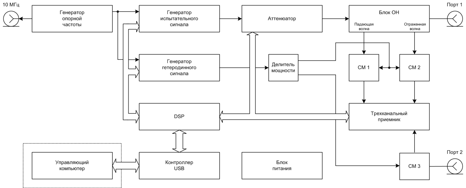
Рисунок 2.1 Функциональная схема анализаторов
