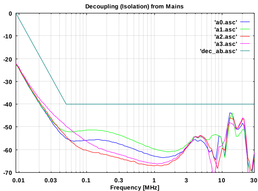
Abb. 9 Entkopplung vom Speisenetz (CEKON-Prüflingsklemmen), BNC mit 50 \Omega Abschluss Decoupling from supply net (CEKON), BNC terminated with 50 \Omega
