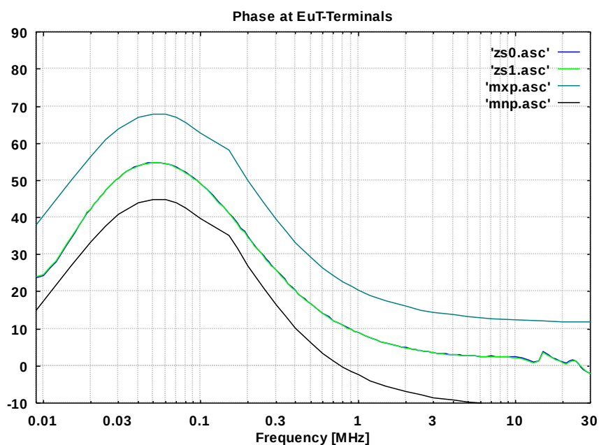
Abb. 8 Phase an den Prüflingsklemmen (SCHUKO), BNC mit 50 \Omega Abschluss Phase at the connector for DuT (Schuko), BNC terminated with 50 \Omega
