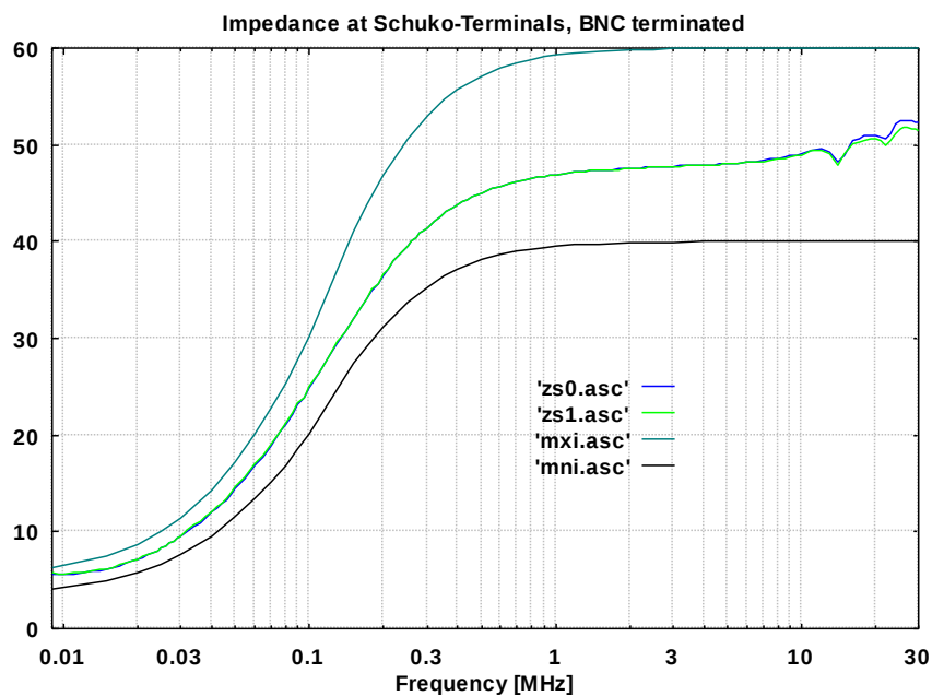
Abb. 7 Impedanz an den Prüflingsklemmen (SCHUKO), BNC mit 50 \Omega Abschluss Impedance of connector for DuT (Schuko), BNC terminated with 50 \Omega
