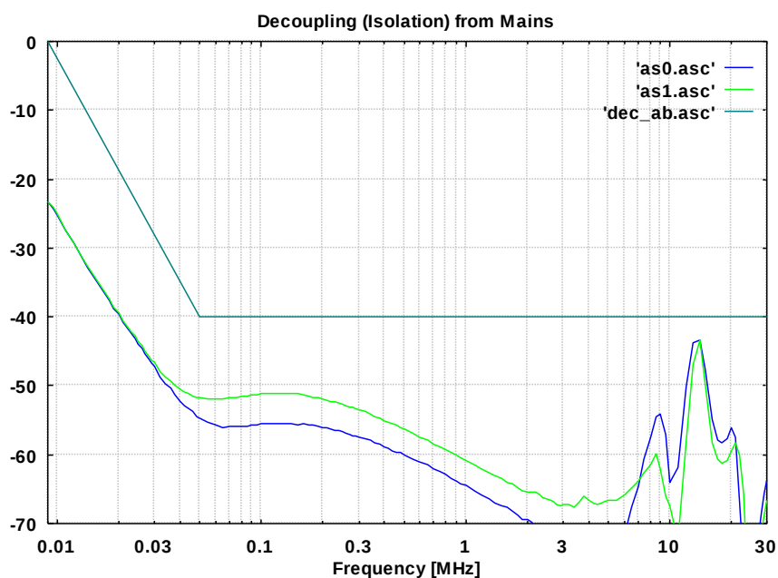
Abb. 10 Entkopplung vom Speisenetz (SCHUKO-Prüflingsklemmen), BNC mit 50 \Omega Abschluss/ Decoupling from supply net (Schuko), BNC terminated with 50 \Omega
