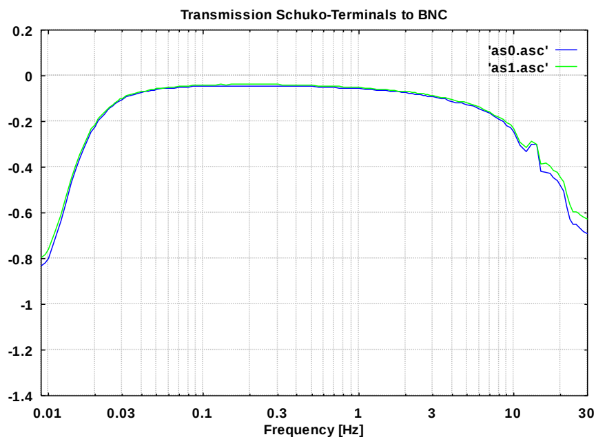
Abb. 6 Transmission Prüflingsklemmen Schuko – BNC Transmission Schuko - BNC
