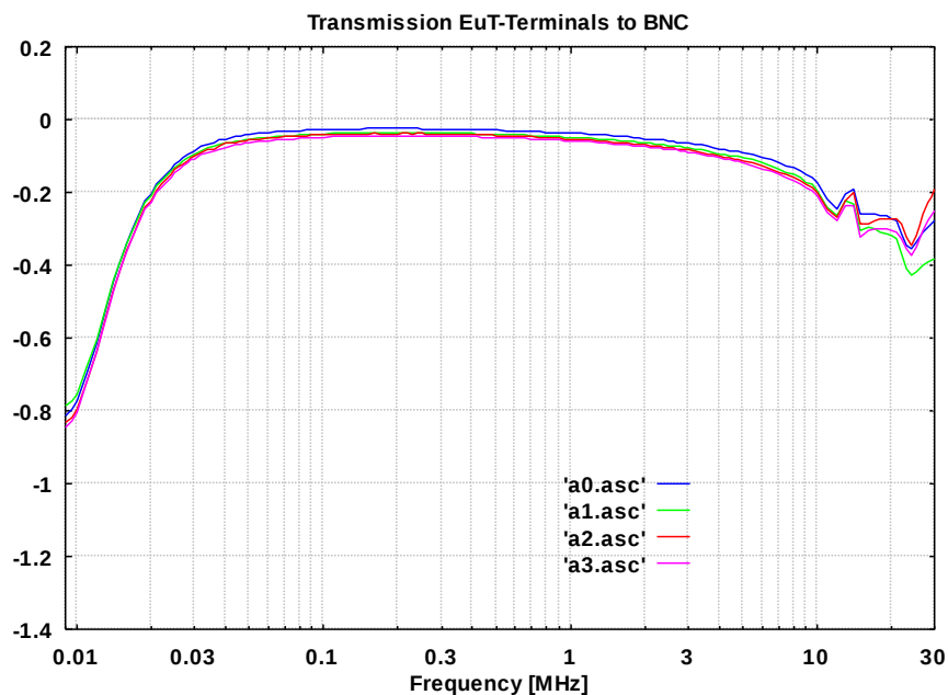
Abb. 3 Transmission Prüflingsklemmen (CEKON) - BNC Transmission CEKON - BNC
