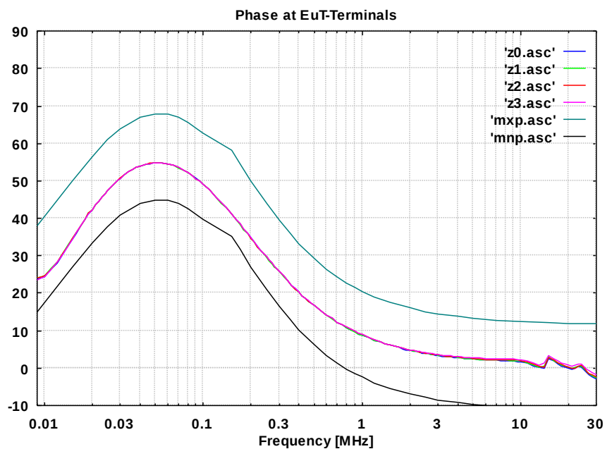
Abb. 5 Phase an den Prüflingsklemmen (CEKON), BNC mit 50 \Omega Abschluss Phase at the connector for DuT (CEKON), BNC terminated with 50 \Omega
