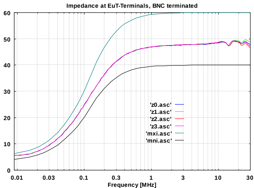
Abb. 4 Impedanz an den Prüflingsklemmen (CEKON), BNC mit 50 \Omega Abschluss Impedance of connector for DuT (CEKON), BNC terminated with 50 \Omega
